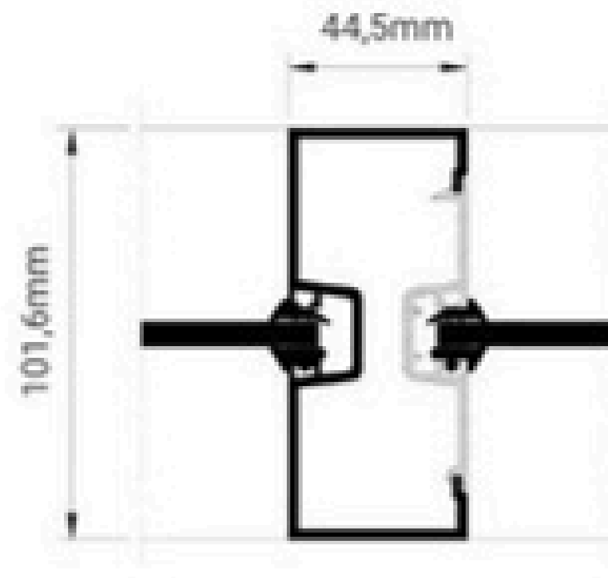
Vertical típico
