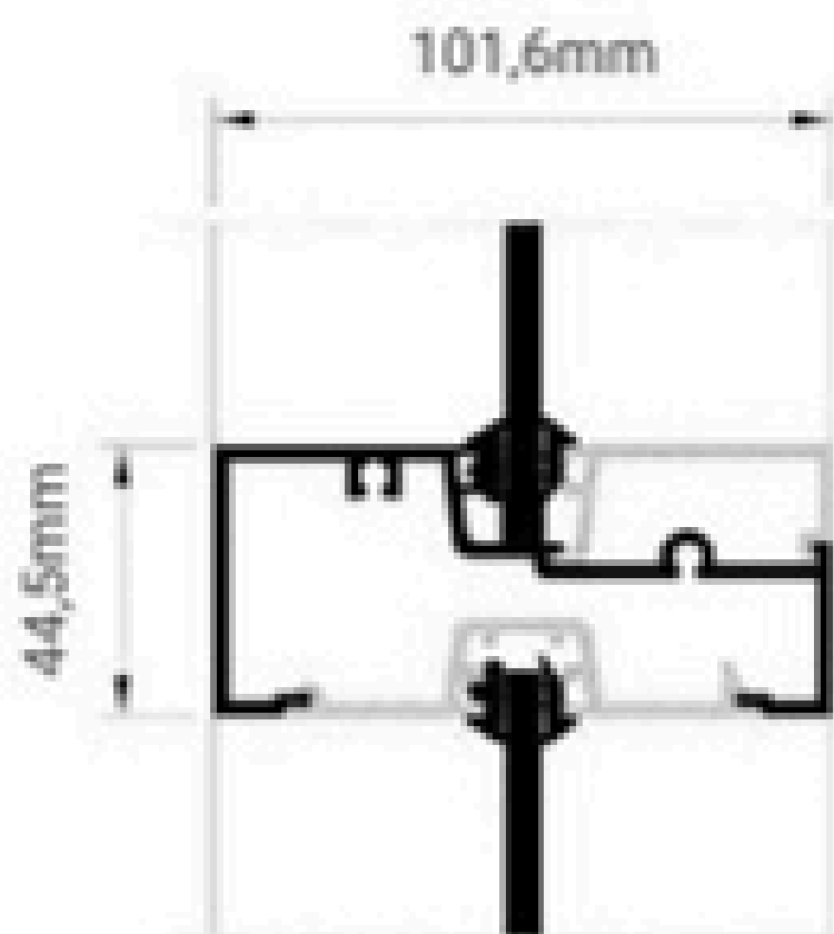
Horizontal típico
